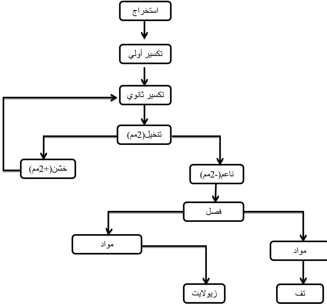
رسم توضيحي 3 : وصف العملية الإنتاجية
